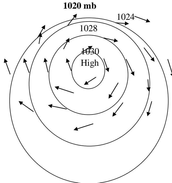
Fig. 11 : Anticyclone
