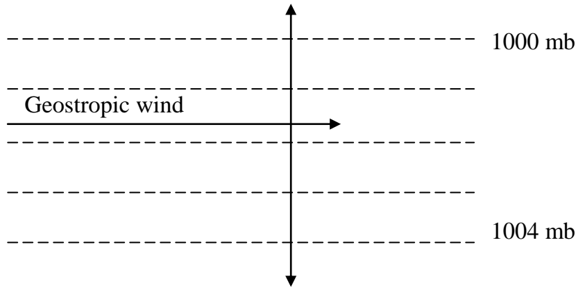
Fig 5 : Geostropic wind
