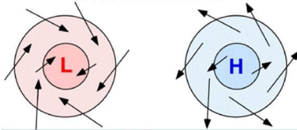
Fig. 8 : Cyclone
